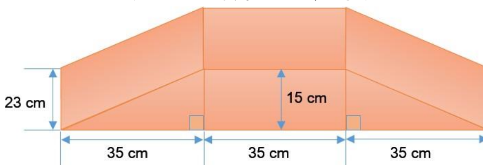
圖B：終點爬坡平臺規格尺寸示意圖
