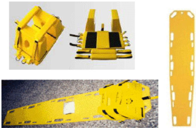
圖五 軀幹固定器
